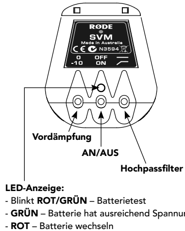
Abb. 7 – Rückseite des Stereo VideoMic
