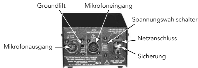
Abb. 1 – Rückseite des NTK-Netzteils
