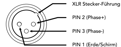
Abb. 5 – XLR-Anschluss
