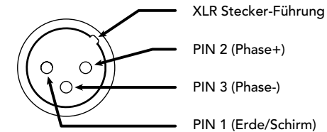
Abb. 3 – XLR-Anschluss
