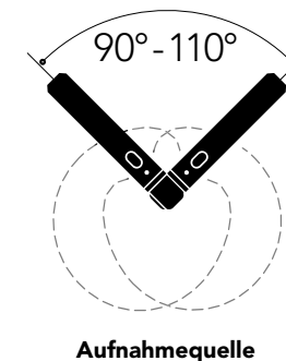
Abb. 8 – XY-Mikrofonie
