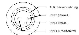
Abb. 4 – XLR-Anschluss
