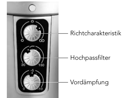
Abb. 3 – Drehregler des NT2000
